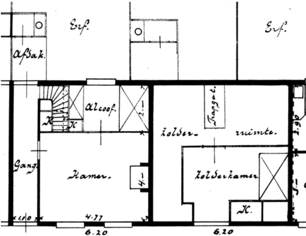
De oude plattegrond van een tussenwoning, het meest voorkomende type in de Hollanderwijk. Een deel van de woningen werd gespiegeld. Op de verdieping is een slaapkamer afgetimmerd, met een vast bed en een opbergkast.
