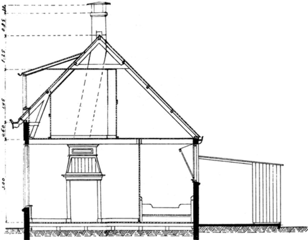
Op de doorsnede is de schouw te zien, het alkoof (met bed en klpraam), het 'werkplaatsje' onder het afdak en het 'privaat'.
